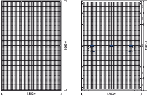
ÖN GÖRÜNÜŞ
